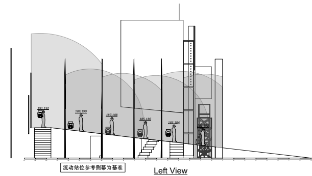
流动站位参考侧幕为基准
