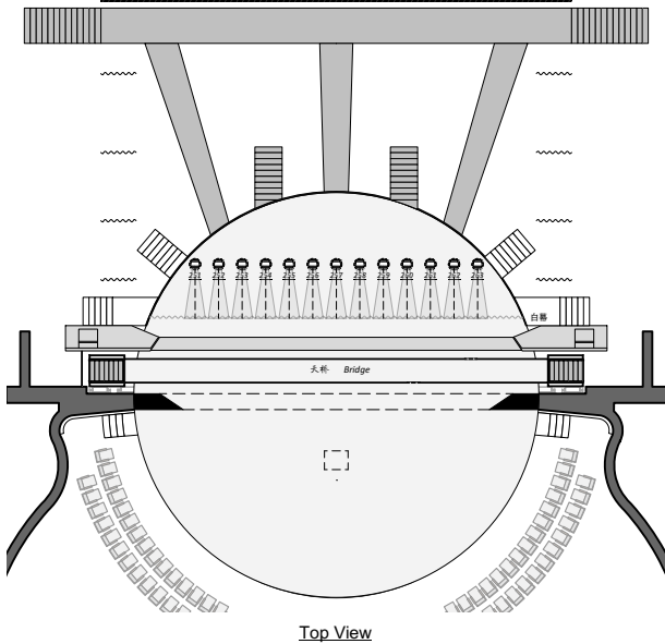
Electric #4 13 - Claypaky BeeEye K20 使用最小光斑角投射到白幕后，反射到环形天幕
